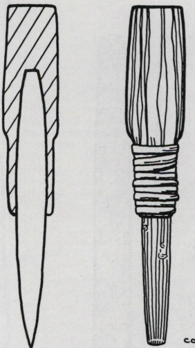
Fig. 3. Forslag til skæftning af fundets mejsler. (Tegnet af Catharina Oksen).
