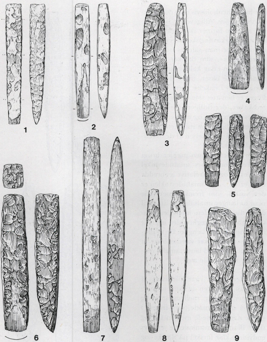
Fig. 4. Bondestenalderens mejseltyper: 1. Kileformet retmejsel (fra Anhoje-depotet, Stevns). 2. Buttet hulmejsel (fra Killerup-jættestuen, Lolland). 3. Tosidet mejsel (fra Karleby, Nordjylland). 4. Spidsnakket hulmejsel (fra megalitgrav ved Bejstrup, Nordjylland). 5. Genbrugsmejsel (fra »Knoldhøj«-jættestuen, Sydsjælland). 6. Kileformet hulmejsel (fra offerfund i Værebros Å, Sjælland). 7. Dobbeltmejsel (fra Ringseballe, Lolland). 8. Buttet retmejsel (fra Killerup-jættestuen, Lolland). 9. Tyk retmejsel (fra enkeltgrav ved Koldkur, Midtjylland). (Alle tegnet af H. Ørsnes, 2:5).
